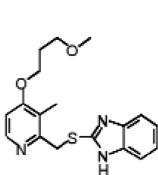
Sulphide
